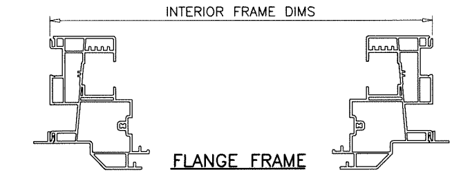
FLANGE FRAME
